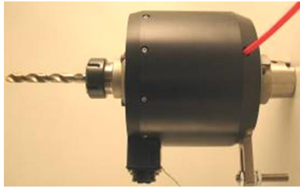
Fig. 3. Rotation free linear actuator
