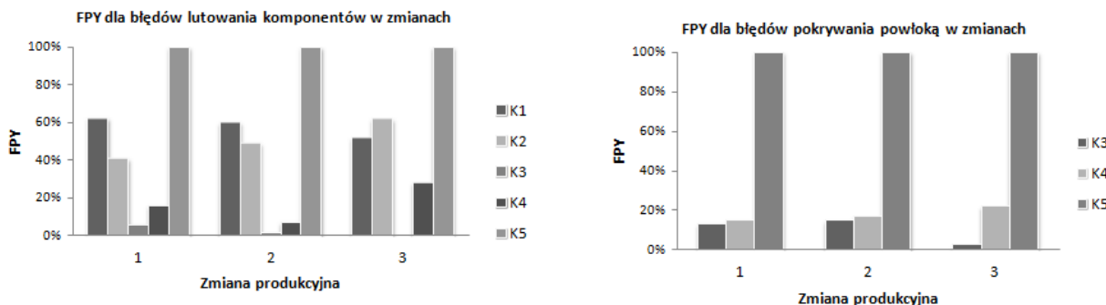
Rys. 5. Wartość wskaźnika FPY dla niezgodności o znanych lokalizacjach w procesie lutowania i oraz o nieznanej lokalizacji w procesie pokrywania powłoką ze względu na zmianę produkcyjną
