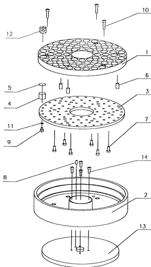
Rys. 9. Konstrukcja narzędzia – wersja II
