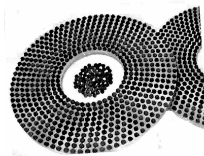
Rys. 4. Konstrukcja tabletkowych narzędzi klejonych [18]
