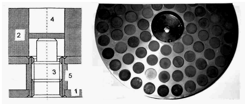
Rys. 8. Konstrukcja narzędzia – wersja I
