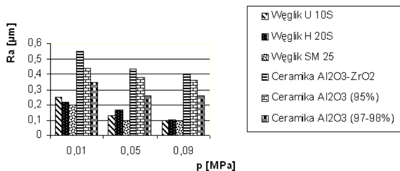
Rys. 15. Chropowatości powierzchni elementów z węglików spiekanych i ceramiki Al 2 O 3 -ZrO 2 (docierak ścierno-metalowy, V=40,7m/min, n=4, t=8min) Fig. 15. Surface roughness of sintered carbides and Al 2 O 3 -ZrO 2 ceramic parts (abrasive-metallic tools, V=40.7m/min, n=4, t=8min)
