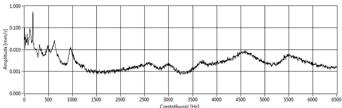
Rys. 7. Częstotliwości drgań wyznaczone w oparciu o transformatę Fouriera dla strugi wodnej
