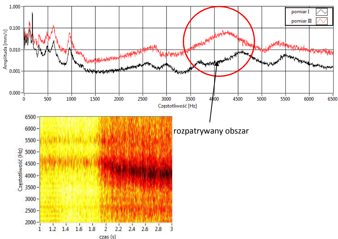
Rys. 8. Porównanie częstotliwości drgań wyznaczonych w oparciu o transformatę Fouriera dla przepływu strugi czystej wody i strugi wodnej ze ścierniwem oraz rozkład Gabora ujmujący moment włączenia ścierniwa
