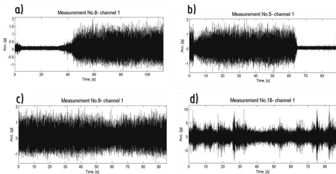
Rys. 6. Przykładowe zapisy rejestracji przyspieszeń drgań na korpusie łożyska kruszarki
