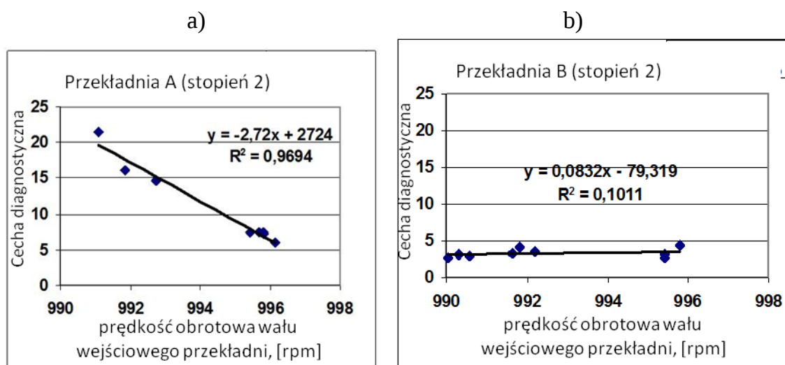
Rys. 7. Zależność wartości cech diagnostycznych od prędkości obrotowej dla przekładni zębatej w stanie:
