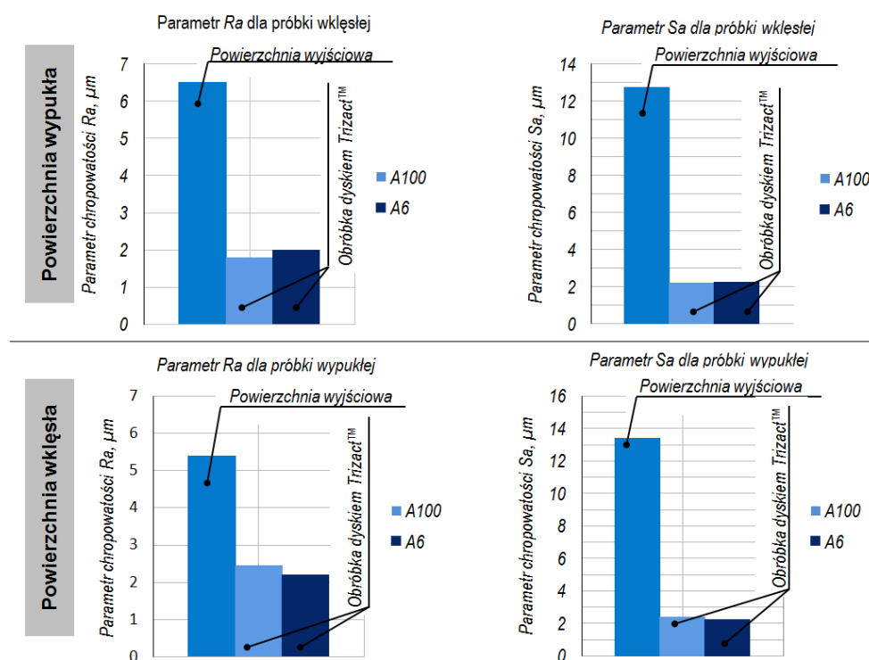
Rys. 10. Wartość średnia z pięciu pomiarów chropowatości powierzchni wklęsłej oraz wypukłej po wygładzaniu dyskami ściernymi Trizact™ o zróżnicowanej gradacji: a) parametr Ra , b) parametr Sa
