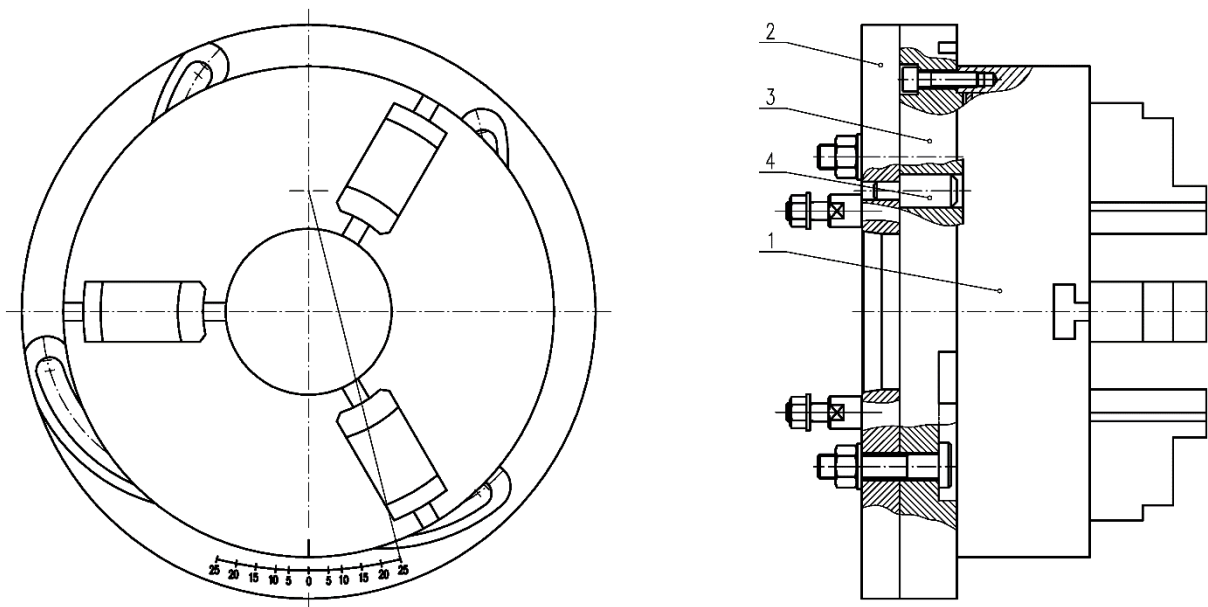
Rys. 4. Wielopozycyjny przyrząd wychylny do obróbki części mimośrodowych: 1 – uchwyt tokarski, 2 – tarcza zabierakowa 3 – tarcza pośrednicząca, 4 – kołek ustalający Fig. 4. The multi-position production jig for eccentric workpieces: 1 – lathe chuck, 2 – catch plate, 3 – intermediate plate, 4 – dowel pin
