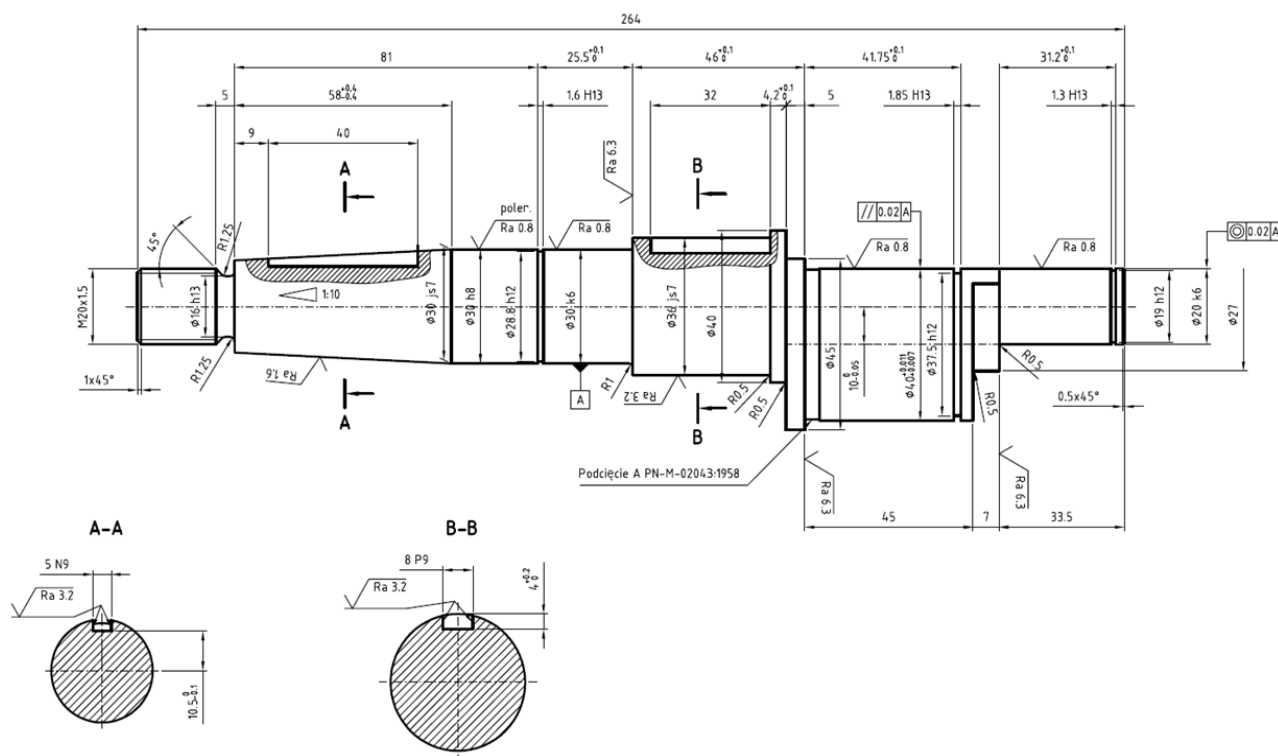
Rys. 7. Wałek mimośrodowy skrzynki grzebieniowej Fig. 7. The eccentric shaft of comb box
