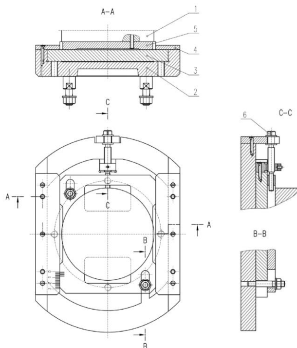
Rys. 2. Wielopozycyjny przyrząd przesuwny z naciętym noniuszem: 1 – uchwyt tokarski, 2 – tarcza, 3 – przeci ciężar, 4 – prowadnice, 5 – płyta uchwytu, 6 – śruba specjalna
