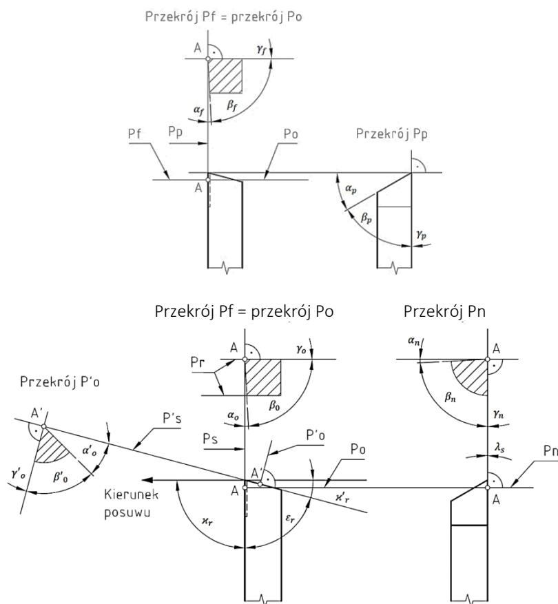
Rys. 8. Kąty ostrza noża tokarskiego w roboczym układzie odniesienia: \alpha_p=30^\circ , \gamma_p=0^\circ , \beta_p=60^\circ , \alpha_f=\alpha_o=3^\circ , \gamma_f=\gamma_o=0^\circ , \beta_f=\beta_o=87^\circ , \alpha'_o=30^\circ , \gamma'_o=0^\circ , \beta'_o=60^\circ , \alpha_n=3^\circ , \gamma_n=0^\circ , \beta_n=87^\circ , K_r=90^\circ , \varepsilon_r=75^\circ , K'_r=15^\circ , r_\varepsilon=0,10 mm, \lambda_s=0^\circ
