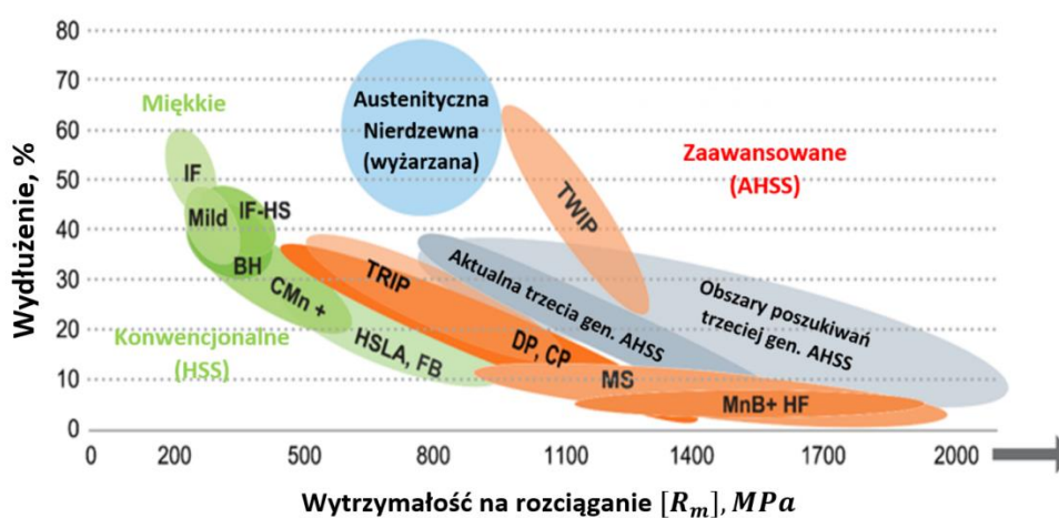
Rys. 2. Właściwości stali przeznaczonych na części nadwozia [3]
